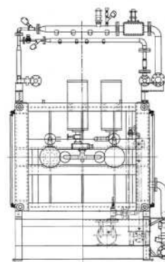
正面图
