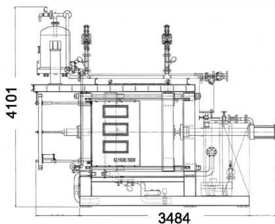
侧面图
