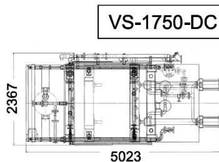
平面图
